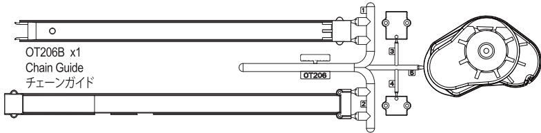
OT205 x1 Holder ホルダー
