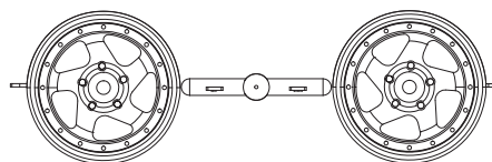
OTH244SC x2 5sp Wheel 43mm Satin Chrome 5スポークホイール43mm(サテンクロームメッキ)
