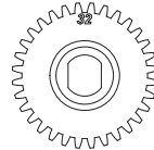
OT221 a x1 Final Pinion Gear 32T ファイナルピニオンギヤ
