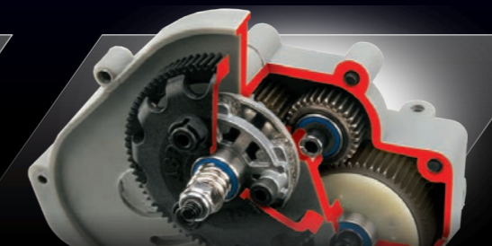
Torque-Control™ Slipper Clutch
