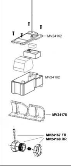
Exploded Diagram Blackout MT Vue éclatée Blackout MT Explosionszeichnung Blackout MT Diagrama desplegado Blackout MT
