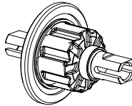
500405867 Centerdiff complete Mitteldiff komplett
