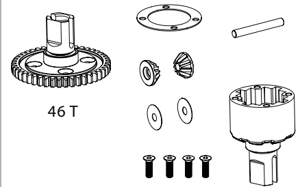
500405592 Centerdiff complete Mitteldiff komplett
