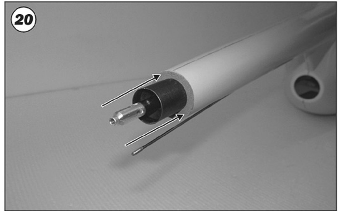
20 Insert a tail boom guide to the tail boom. 將尾管固定環套入尾管。
