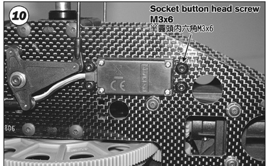
10 Fasten the ELEV servo poles with socket button head screws M3x6. 以半圓頭內六角螺絲M3x6，將固定柱鎖附於側板。
