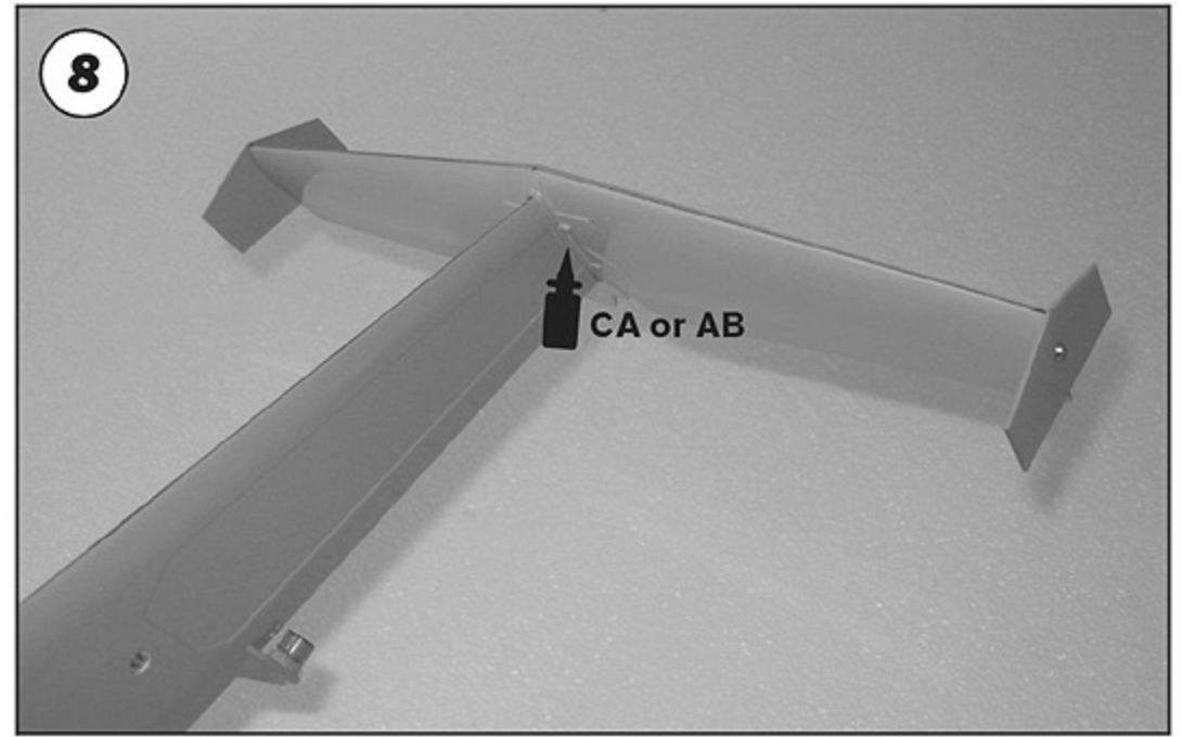
8 Fix the horizontal stabilizer to the vertical stabilizer with CA glue or AB glue. 以CA或AB膠將水平尾翼固定於垂直翼上。
