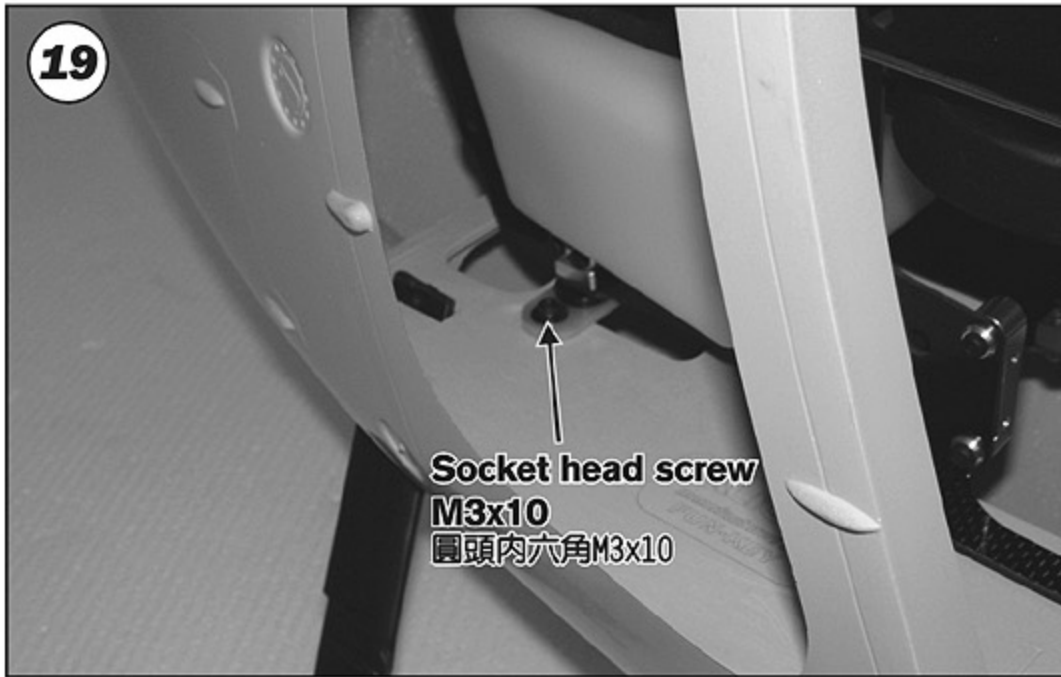
19 Use a hexagon wrench to fasten the fixing plate with socket head screw M3x10 and washer \phi 3.4 \times \phi 9.9 \times \phi 0.9 \text{mm} . 使用L型的六角扳手將圓頭六角螺絲M3x10與華司 \phi 3.4 \times \phi 9.9 \times \phi 0.9 \text{mm} 將固定片鎖緊固定。
